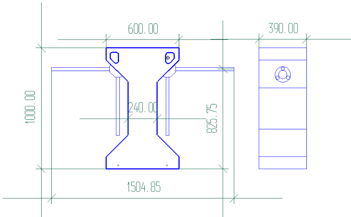
Rys. 4 Gabaryty obudowy
